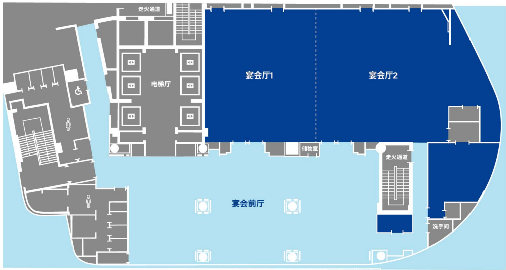
2层平面图
